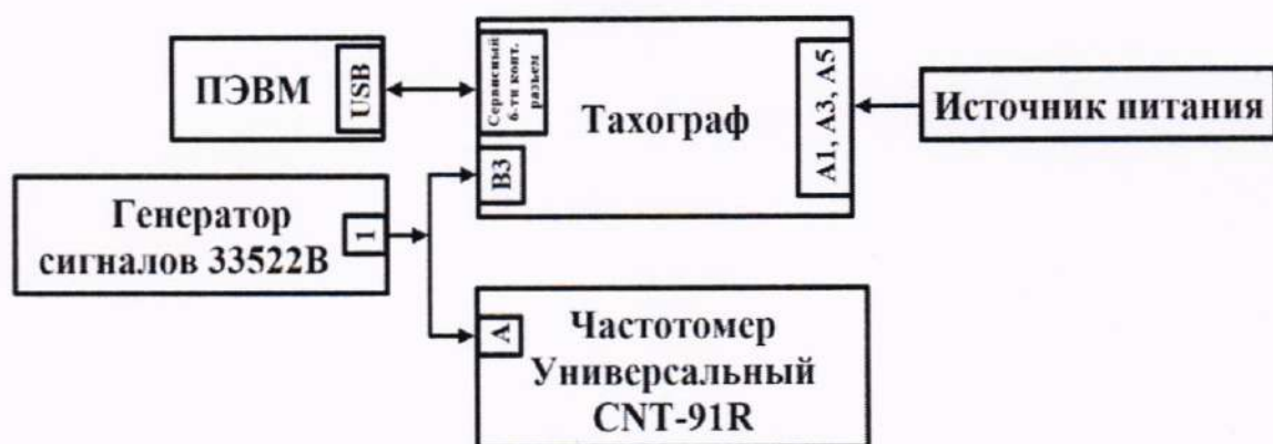
Рисунок 4 – Схема проведения измерений при определении относительной инструментальной погрешности измерений пройденного пути
