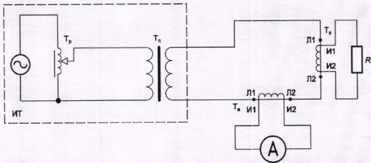
ИТ — регулируемый источник синусоидального тока; — — сеть (генератор); Т р — регулирующее устройство (автотрансформатор); Т н — понижающий силовой трансформатор; Т х — проверяемый трансформатор; Т в — вспомогательный трансформатор; R — резистор
