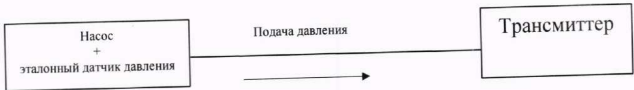
Рисунок 2 – Структурная гидравлическая схема подключения трансмиттера
