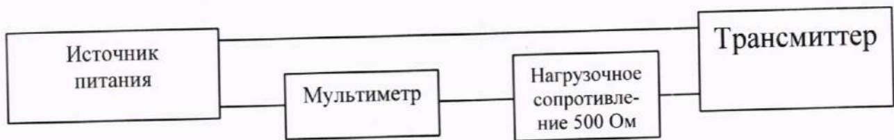
Рисунок 1 – Структурная электрическая схема подключения трансмиттера
