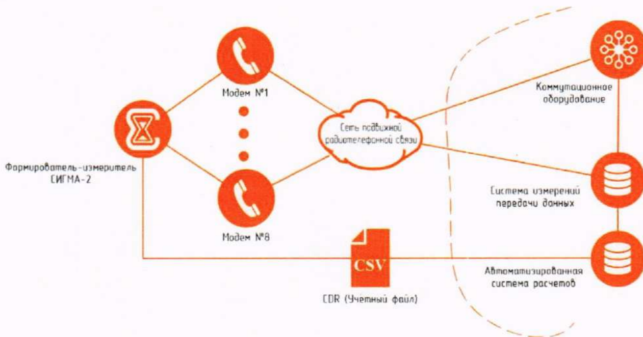
Рисунок 2 – Схема поверки СИПД
