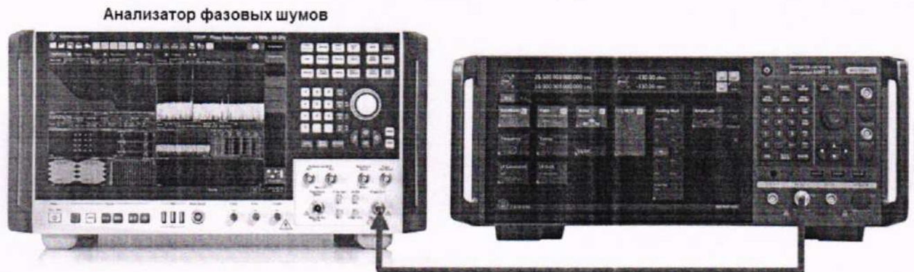
Рисунок 5 – Схема подключения для измерения фазовых шумов с помощью анализатора фазовых шумов FSWP26
