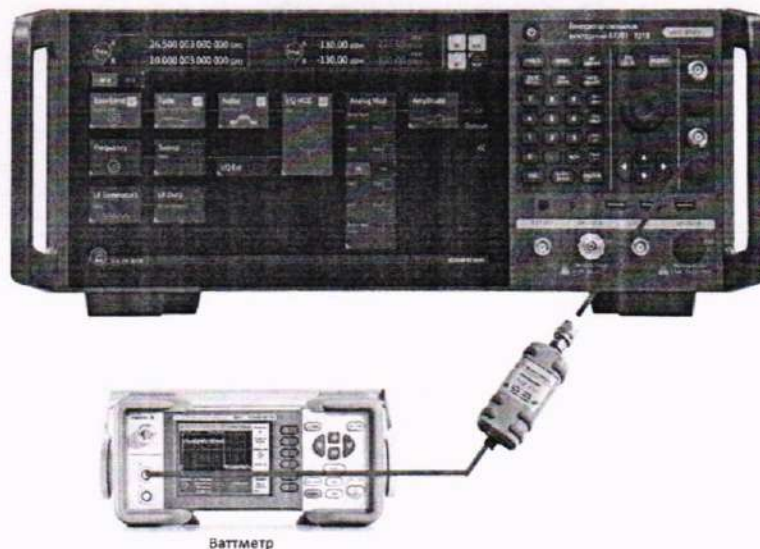
Рисунок 7 – Схема соединения приборов для определения абсолютной погрешности установки размаха синусоидального сигнала
