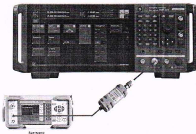
Рисунок 1 – Схема соединения приборов для определения абсолютной погрешности установки максимального уровня выходного сигнала
