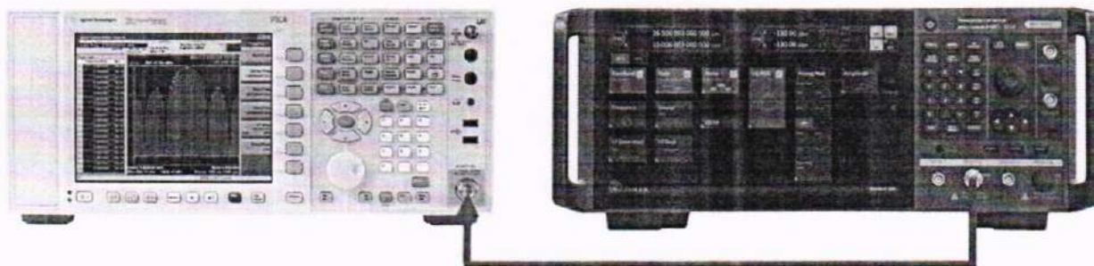
Рисунок 4 – Определение параметров спектра сигнала в режиме непрерывных колебаний
