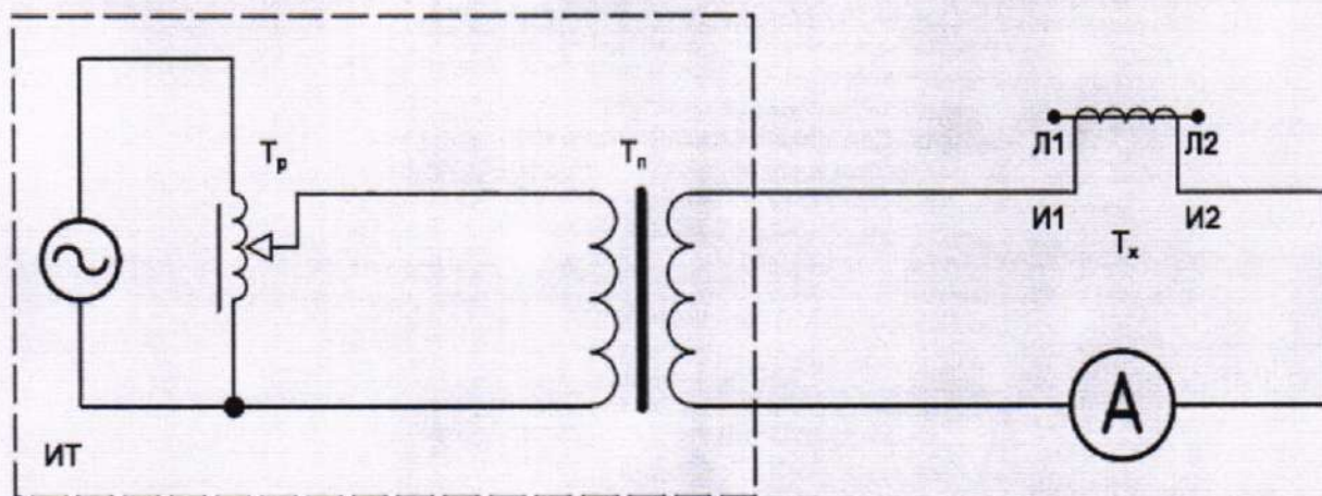
Рисунок 2 – Схема размагничивания трансформатора вторым способом
