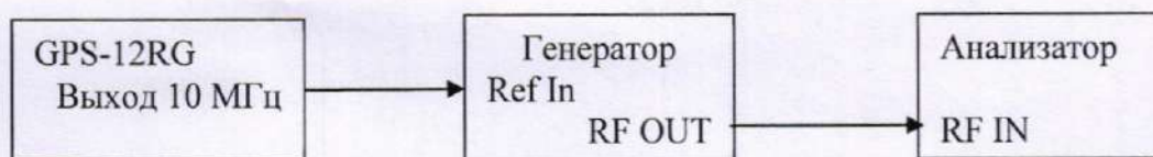
Рисунок 1 – Схема проверки диапазона частот и определения абсолютной погрешности измерений частоты
