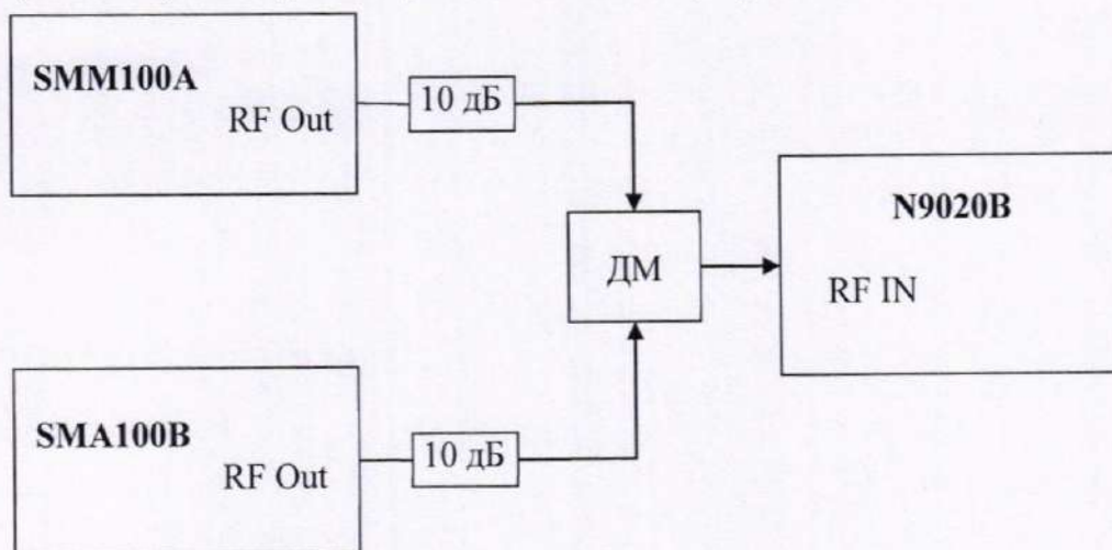
Рисунок 7 – Схема определения относительного уровня помех, обусловленных интермодуляционными искажениями третьего порядка
