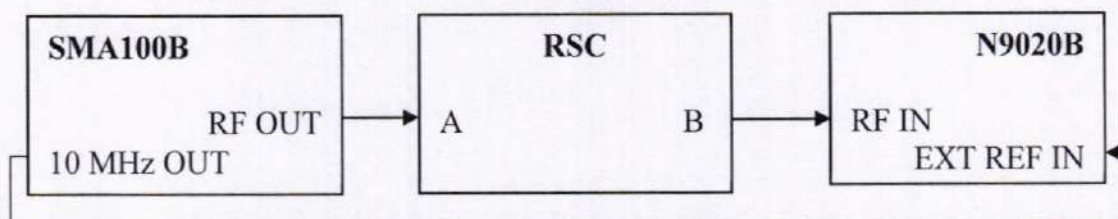
Рисунок 4 – Схема определения неравномерности шкалы дисплея
