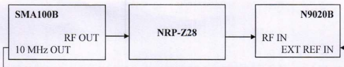
Рисунок 3 – Схема определения абсолютной погрешности измерений мощности
