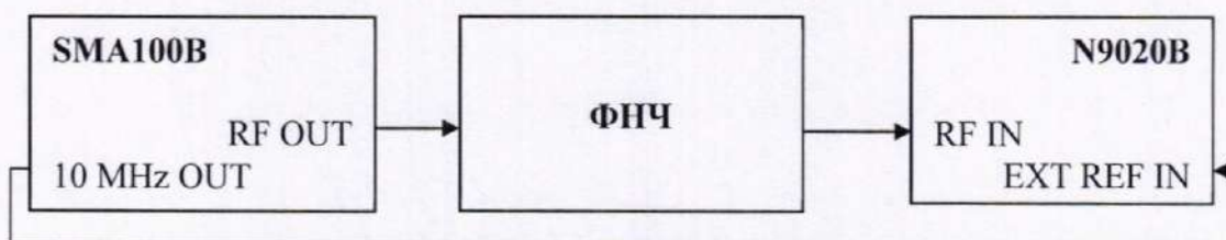
Рисунок 6 – Схема определения относительного уровня помех, обусловленных гармоническими искажениями
