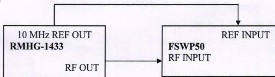
Рисунок 3 – Структурная схема соединения СИ для определения абсолютной погрешности установки уровня мощности выходного сигнала в диапазоне от минимального значения до минус 10 дБ (1 мВт)
