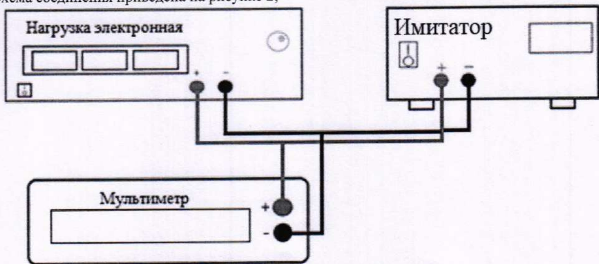
Рисунок 2 – Структурная схема соединения приборов
