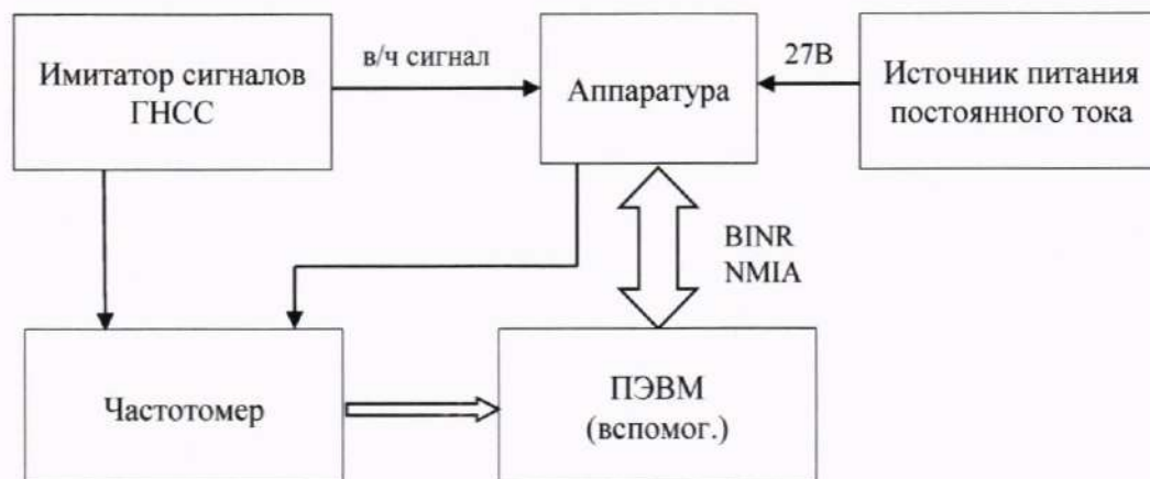
Рисунок 5 - Схема рабочего места по п.10.5
