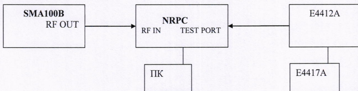
Рисунок 2 – Структурная схема определения относительной погрешности измерений мощности на опорном уровне 1 мВт
