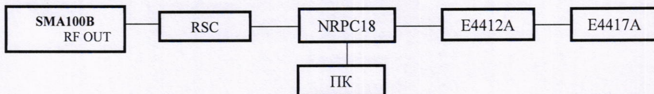
Рисунок 3 – Структурная схема соединения СИ для определения относительной погрешности измерений мощности для уровней мощности минус 70 дБ (1 мВт)
