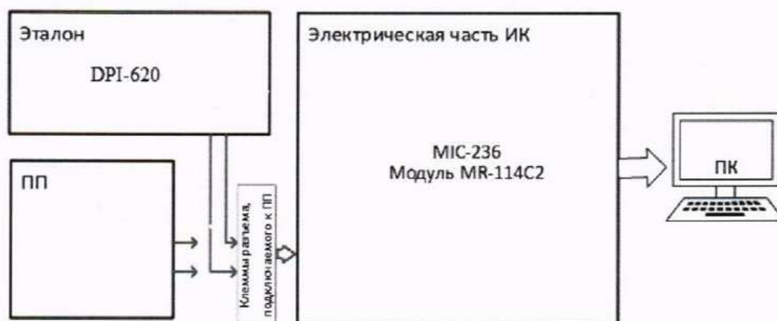
Рисунок 12 – Схема поверки ИК расхода топлива поэлементным способом
