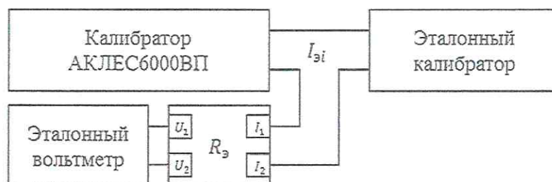
Рисунок 2 – Схема подключения для определения абсолютной погрешности калибратора в режиме измерений силы постоянного тока ( R_э = 100 Ом)
