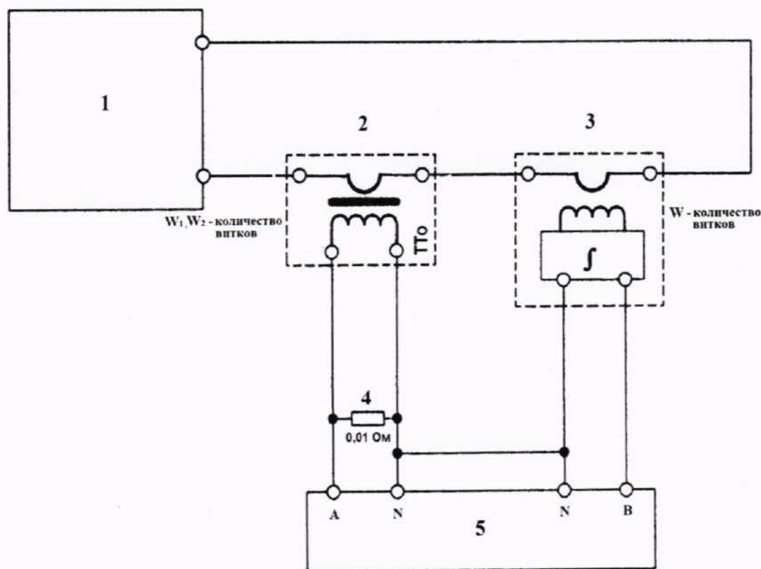
Рисунок 1 - Схема соединений для определения метрологических характеристик
