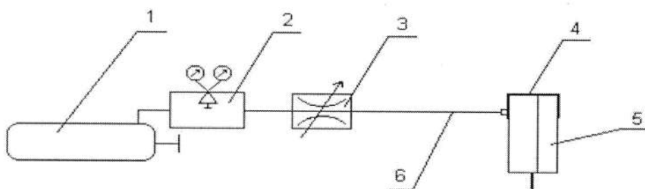
1 - баллон с ГСО-ПГС; 2 - редуктор; 3 - ротаметр; 4 - насадка; 5 - сигнализатор; 6 - трубка ПВХ
