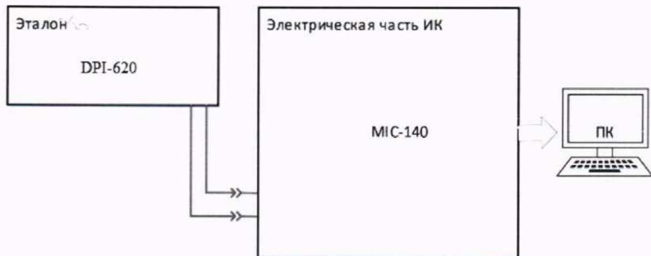
Рисунок 24 – Схема поверки напряжения постоянного тока, соответствующего значениям температуры жидкостей в диапазоне преобразований ПП термоэлектрического типа ТХК (L)
