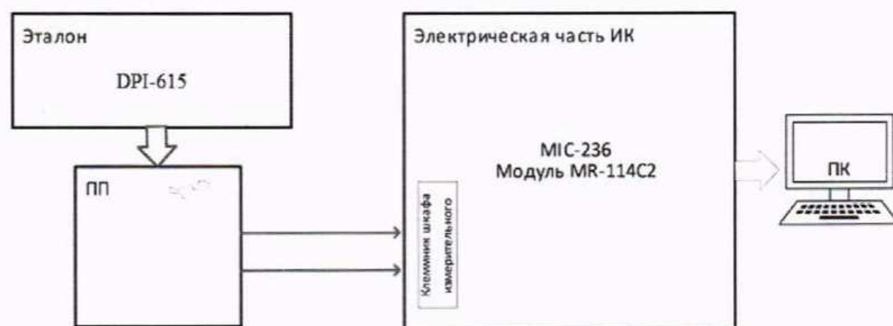
Рисунок 15 – Схема поверки ИК избыточного и разности давлений газообразных и жидких сред
