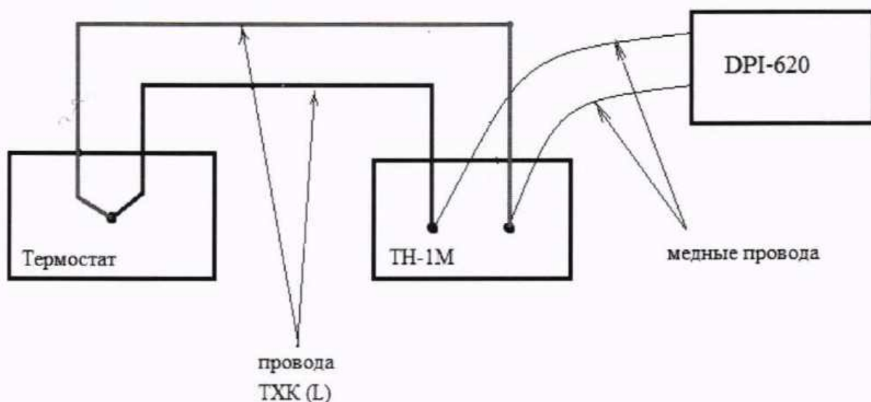
Рисунок 17 – Схема поверки контроля (оценки) ПП для ИК температуры, измеренной ПП термоэлектрического типа ТХК (L)
