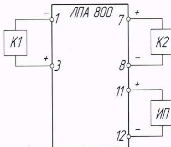
Рисунок А.1 Схема подключения повторителей ЛПА-800-210 и ЛПА-800-200 при опробовании и определении основной приведенной погрешности преобразования силы постоянного тока в значения силы постоянного тока в рабочем диапазоне преобразования
