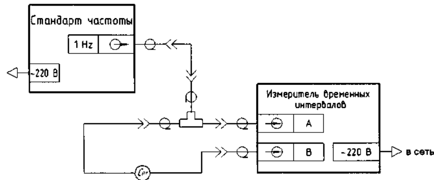
Рисунок А.1 — Схема измерения ГВЗ в коаксиальном кабеле
