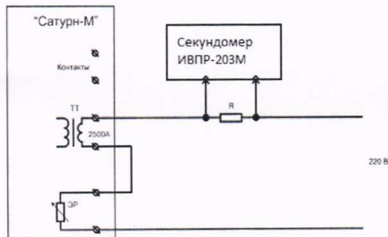
Рисунок 3 - Схема испытаний для определения погрешности измерения длительности протекания тока в цепи
