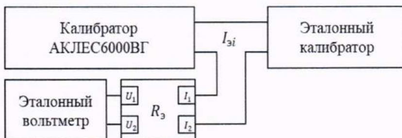
Рисунок 2 – Схема подключения для определения абсолютной погрешности калибратора в режиме измерений силы постоянного тока ( R_z = 100 Ом)
