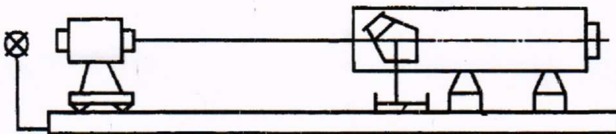
Рисунок 1 – Поверки нивелира на компараторе эталонном
