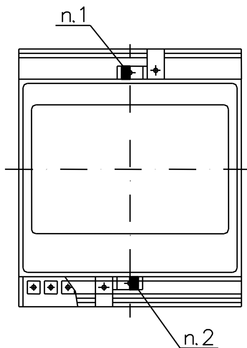
Рисунок 2 - Схема указания мест расположения клейма ОТК (1) и клейма (наклейки) поверителя (2) на преобразователе E855-Ц
