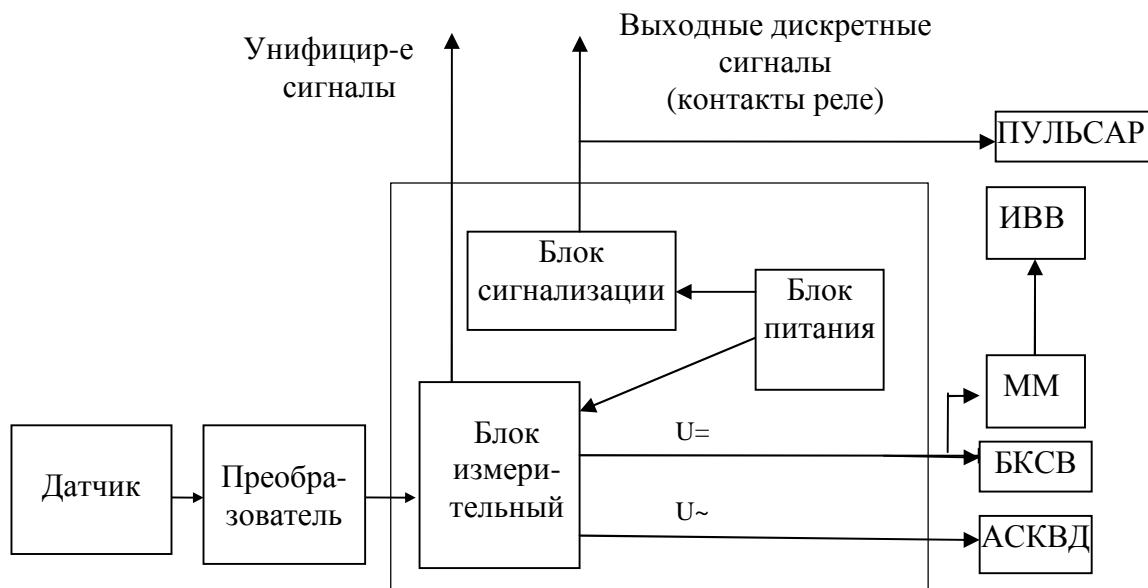
Рисунок 2 - Структурная схема
