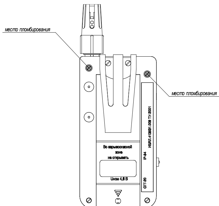
Рисунок 2 - Схема пломбировки сигнализаторов всех исполнений от несанкционированного доступа и обозначение мест для нанесения оттисков клеем
