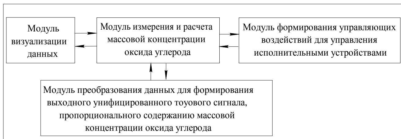
Рисунок 1 - Структура ПО
