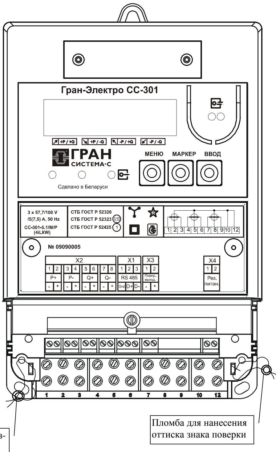
Рисунок 5 – Места клеммения и пломбирования счетчика «Гран-Электро СС-301»
