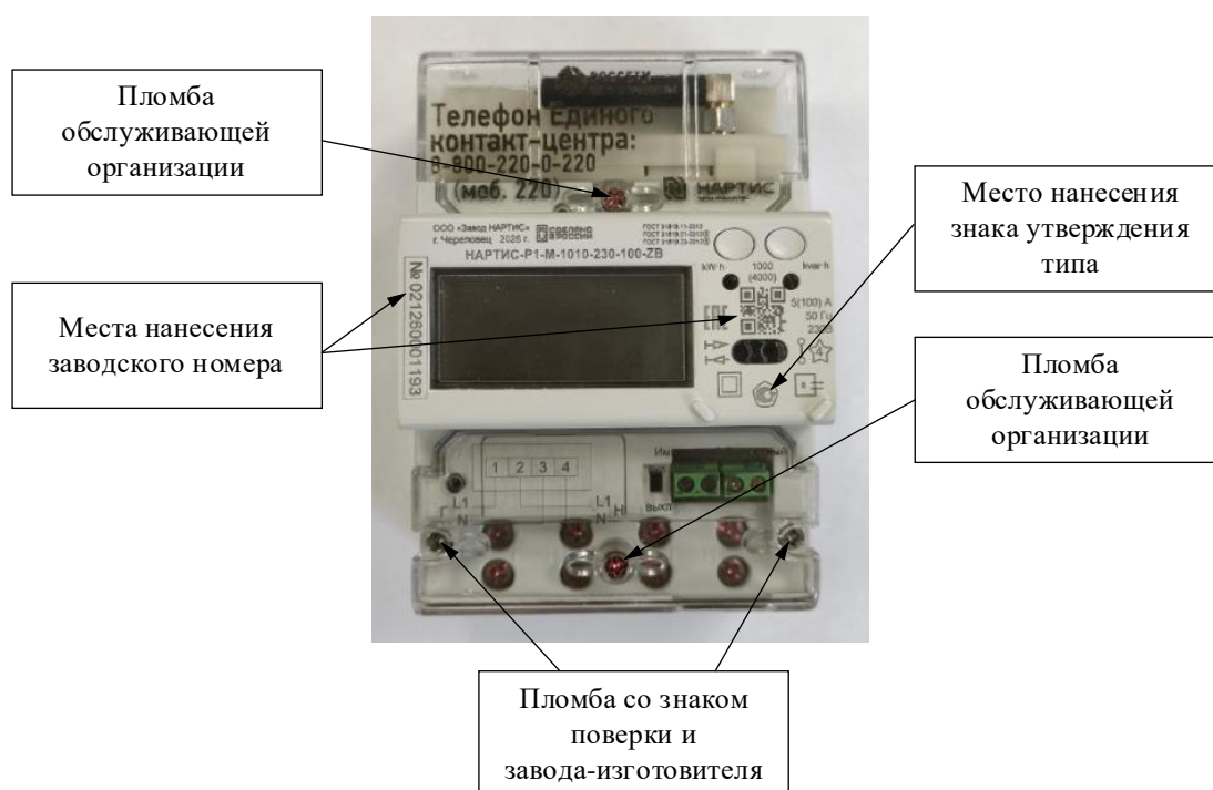
б) счетчики шкафного исполнения НАРТИС-Р1-М
