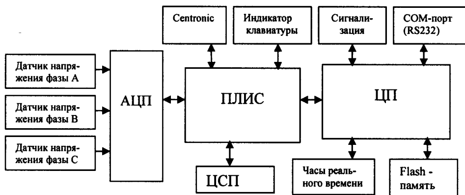
Блок –схема регистратора РК3.01/РК3.01ПТ
