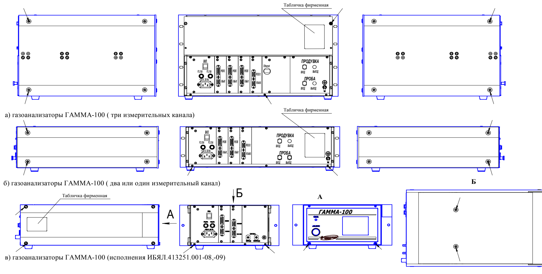
Рисунок 5 - Схема пломбировки газоанализаторов от несанкционированного доступа и обозначение мест для нанесения оттисков клейм
