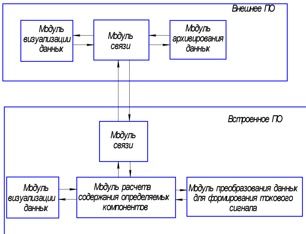
Рисунок 1. Структура ПО.
