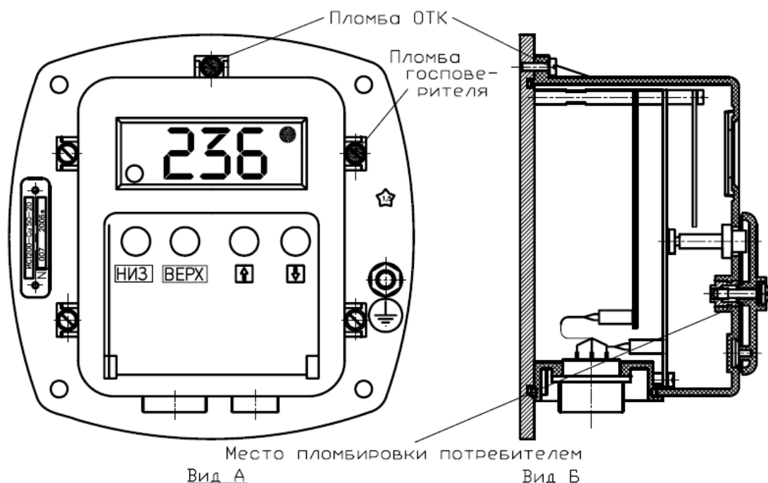
Рисунок 2 – Места пломбирования измерителя-сигнализатора температуры ИСТ Вид А – открытая крышка и органы управления Вид Б – закрытая крышка
