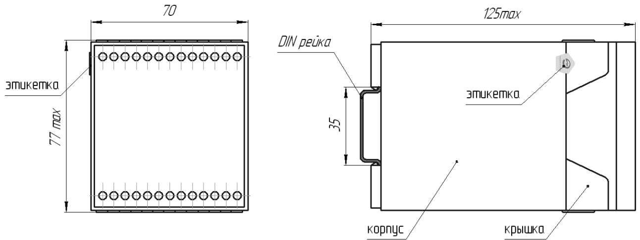
Рисунок 3 – Схема пломбировки от несанкционированного доступа исполнения DIN
