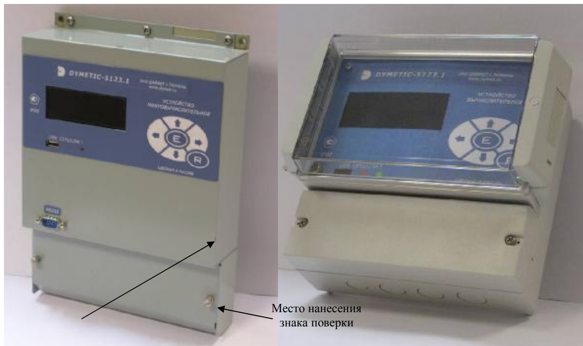
Рисунок 1 – Общий вид вычислителя
