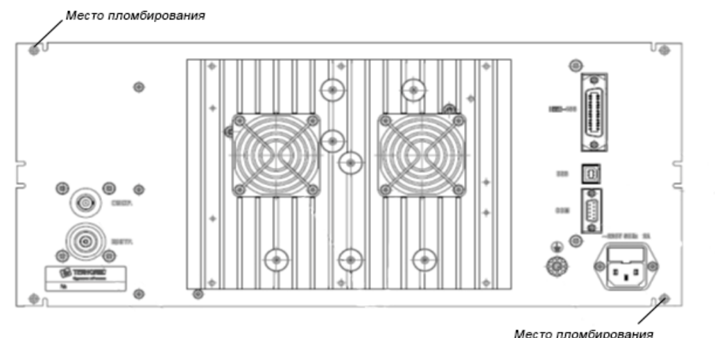
Рисунок 2 - Внешний вид калибратора (вид сзади)
