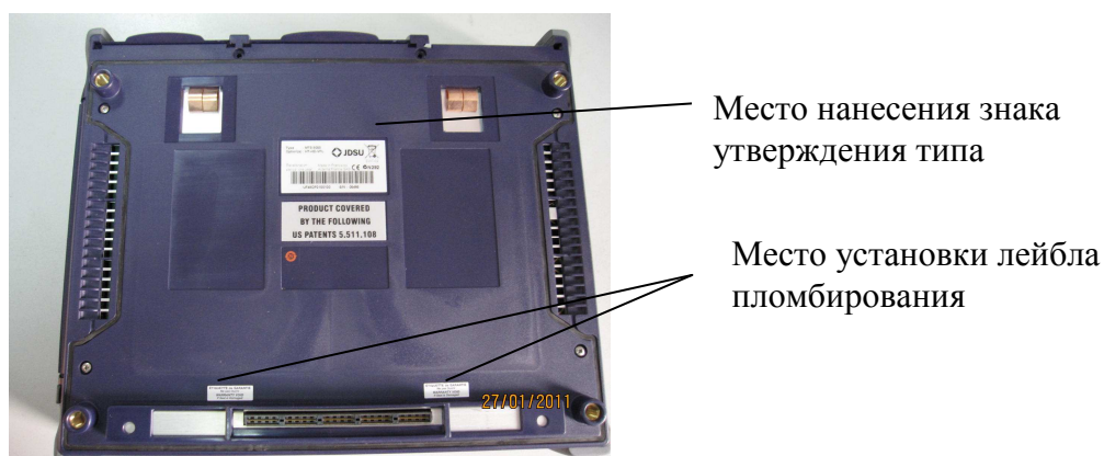
Рисунок 2 - Корпус базового модуля, схема пломбирования
