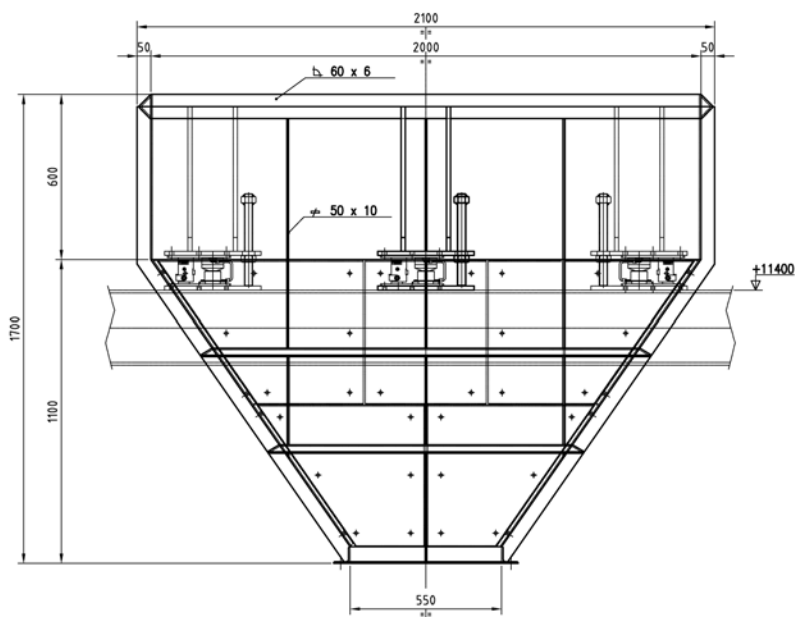
Грузоприемное устройство весов
