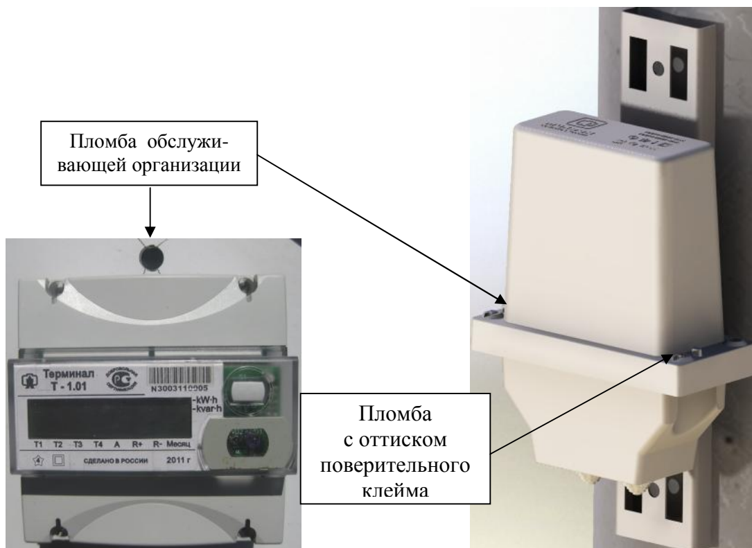
Рисунок 2 – Внешний вид счетчиков наружной установки и схема пломбирования
