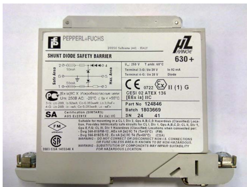
Рис. 1 Фотография общего вида преобразователя измерительного
