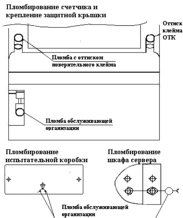
Рисунок 2 – Места установки пломб на технические средства АИИС КУЭ
