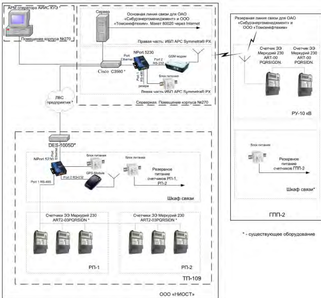
Рисунок 1 – Структурная схема АИИС КУЭ
