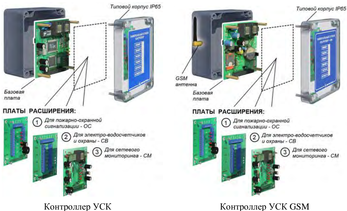
Рисунок 2а. Фотографии общего вида аппаратных средств ПТК «Спрут-М» - контроллеров УСК.
