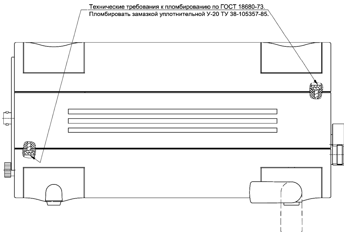
Рисунок 2. Места пломбирования и нанесения поверительных клеем
