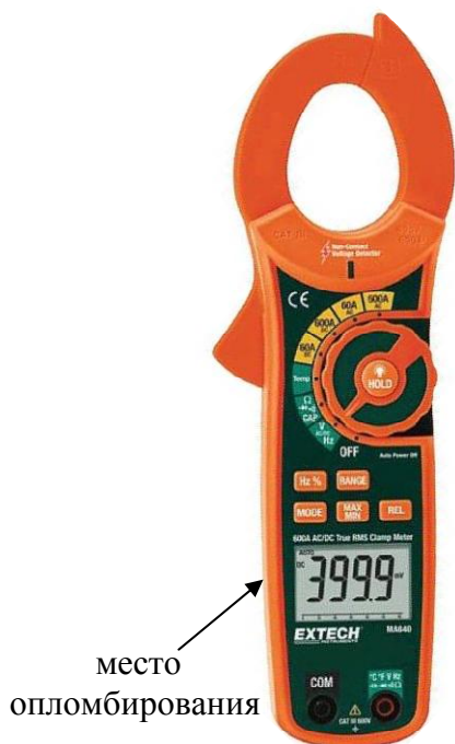
Рисунок 8. Модель MA640
