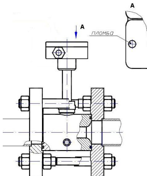
Рисунок 1 – Схема пломбирования датчика расхода газа ДРГ.М-1600
