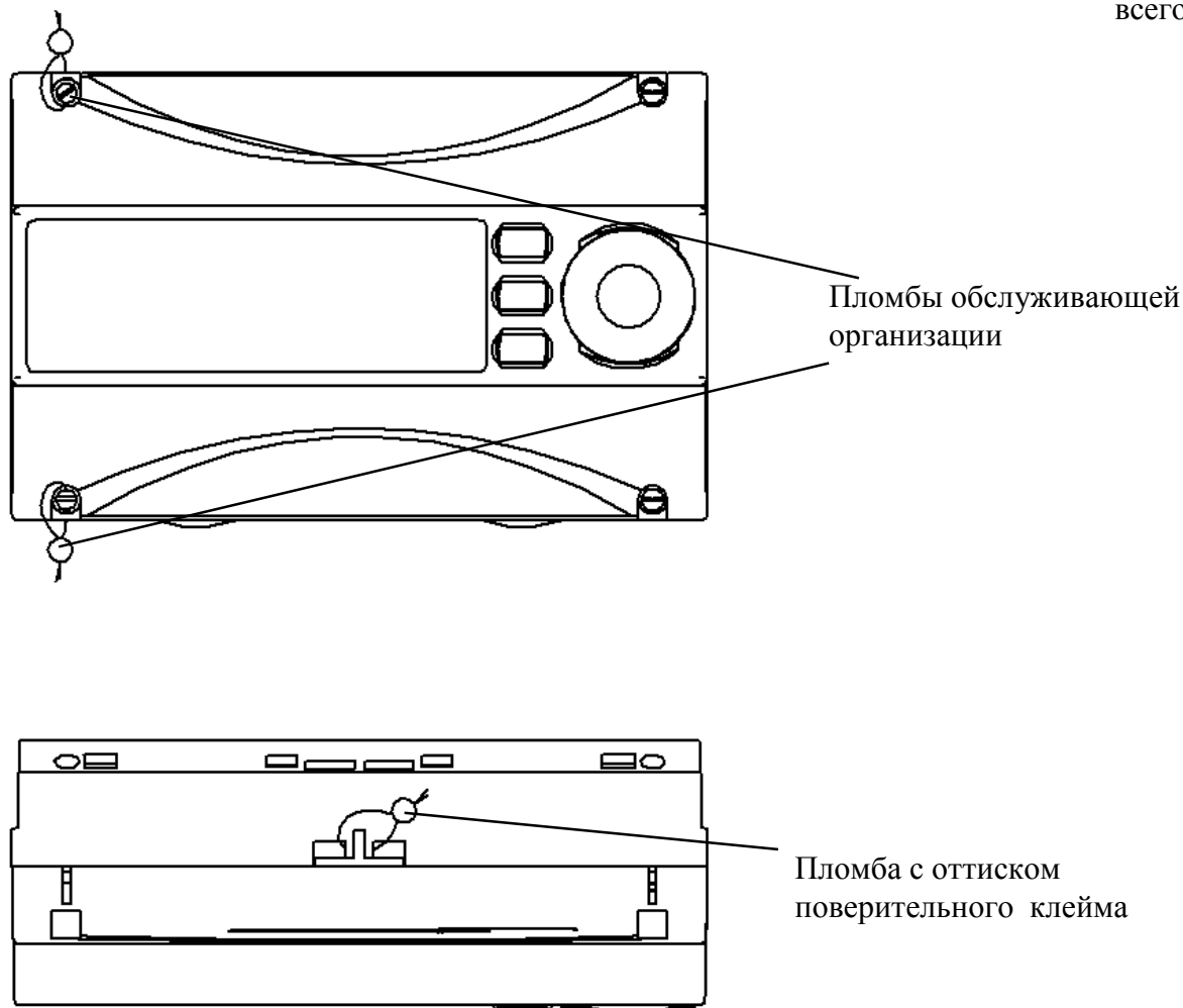
Рисунок 3 – Схема пломбирования счётчика
