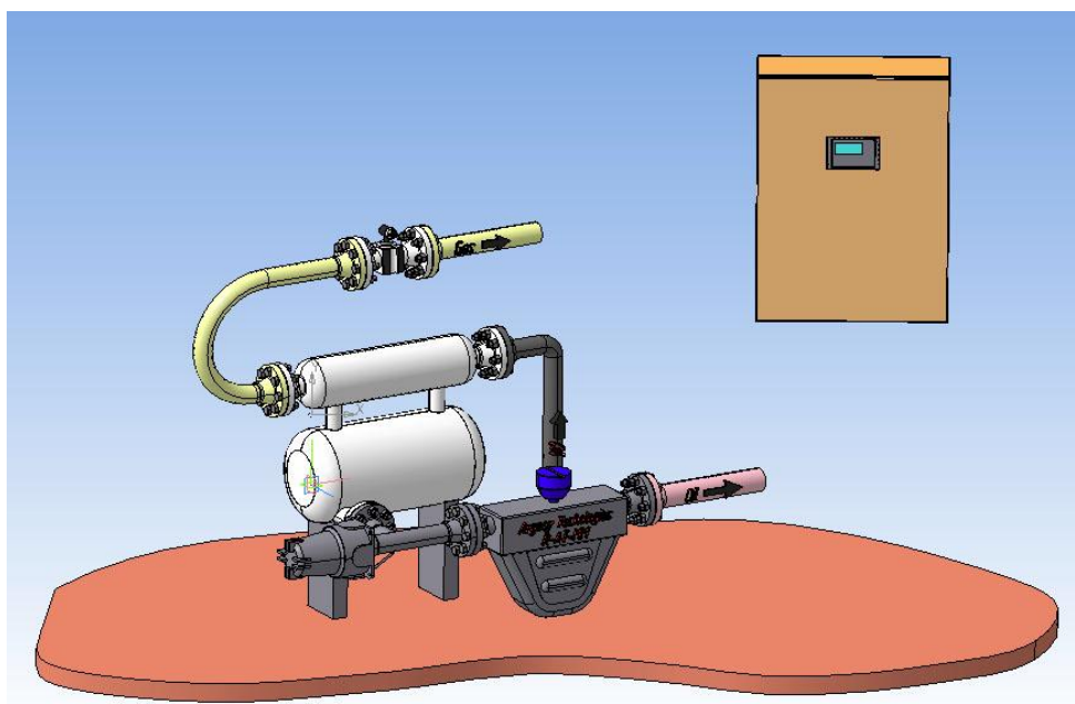
3D изображение измерительной части установки
