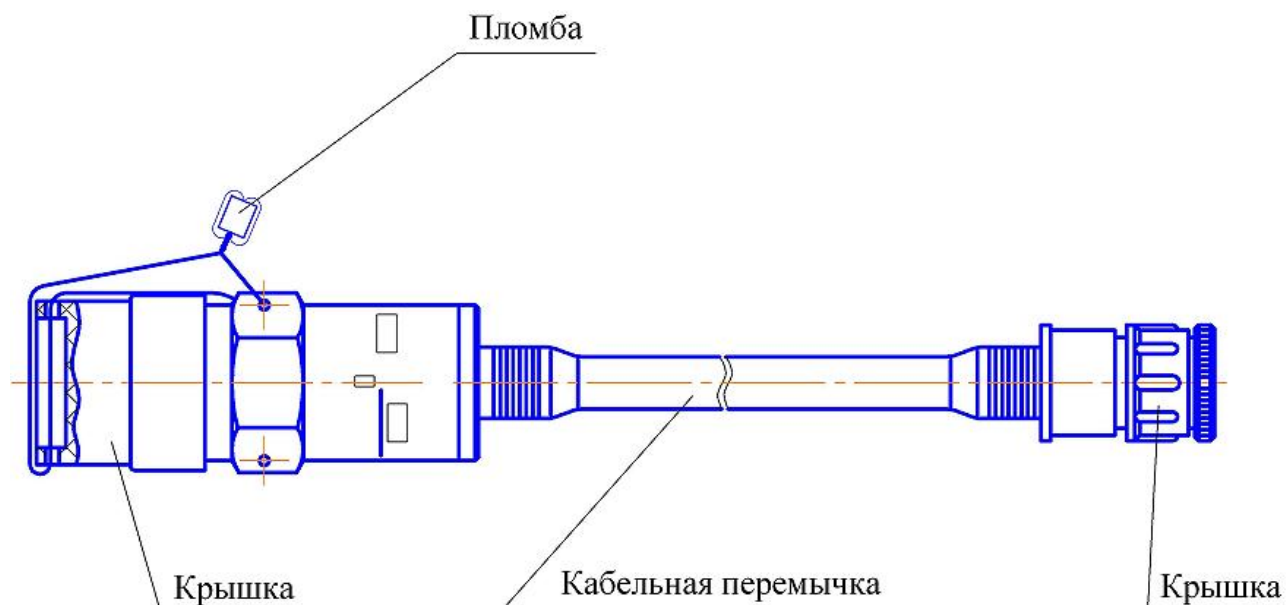
Рисунок 2 - Схема пломбирования от несанкционированного доступа
