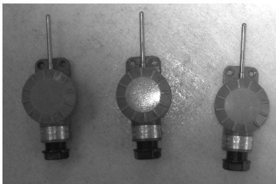
Рис.1 Термопреобразователи сопротивления ТСМ-1290.
