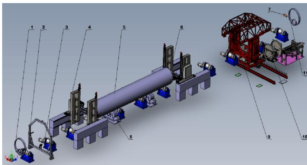
Рисунок 1 – система контроля геометрических параметров труб «МРТ-1420» («MRT-1420»)
