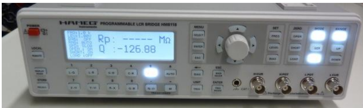
Рисунок 1 – Общий вид передней панели измерителя иммитанса
