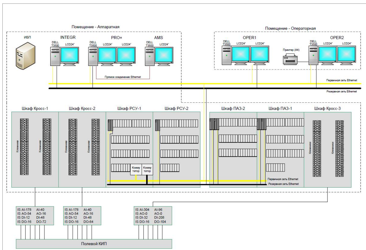
Рисунок 2 – Структурная схема ПТК АСУ ТП СПГК ООО «Афипский НПЗ»
