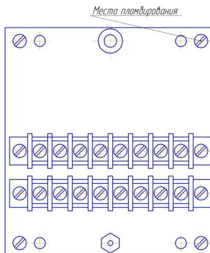
Рисунок 2 Внешний вид и схема пломбирования РТМ-3 щитового исполнения
