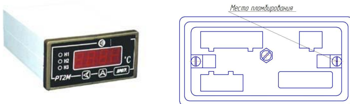
Рисунок 1 Внешний вид и схема пломбирования РТ2М
