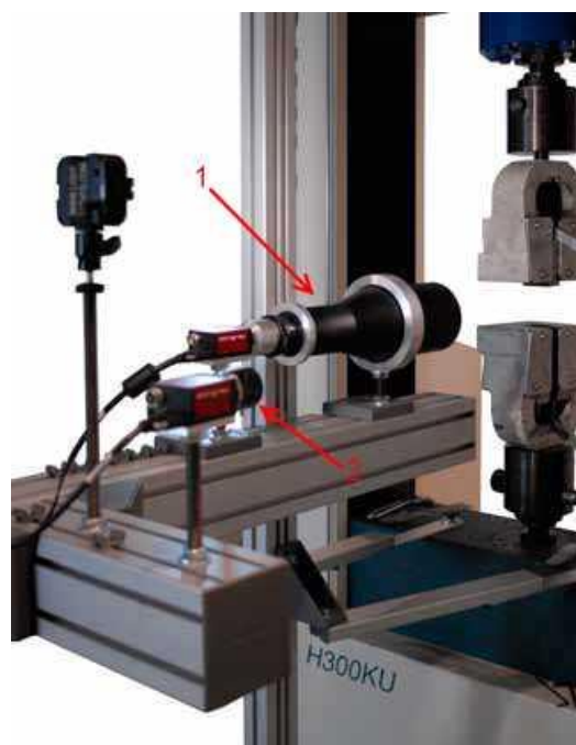
Рис.1 Внешний вид измерителей перемещений (деформаций) бесконтактных VETO
